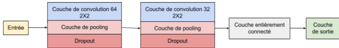
Fig 4.3 Diagramme du modèle d'apprentissage profond utilisé
