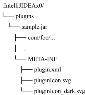
Fig 3.7 Structure de projet d'un plugiciel sans dépendances [28]
