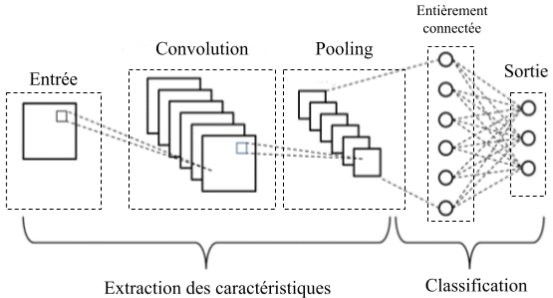
Fig 4.1 Architecture basique des RNC [36]
