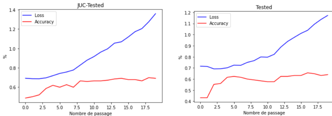
Graphique 5.3 Perte et Précision entre les étiquettes avec le système JFREECHART
