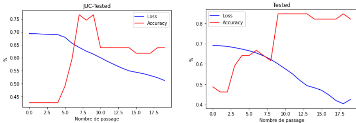
Graphique 5.1 Perte et Précision entre les étiquettes avec le système IO
