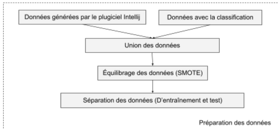
Fig 3.3 Sous-processus dans l'étape de préparation des données
