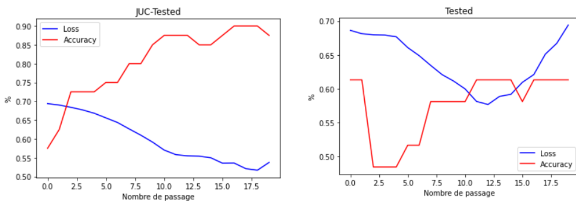
Graphique 5.2 Perte et Précision entre les étiquettes avec le système MATH
