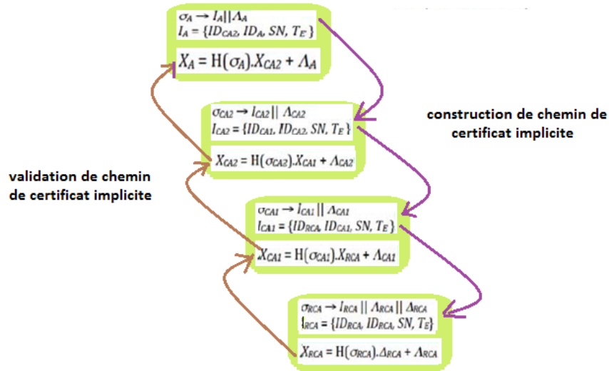
Figure 4 : Construction et validation du chemin de certificat implicite pour SCS basé sur ECC[17]
