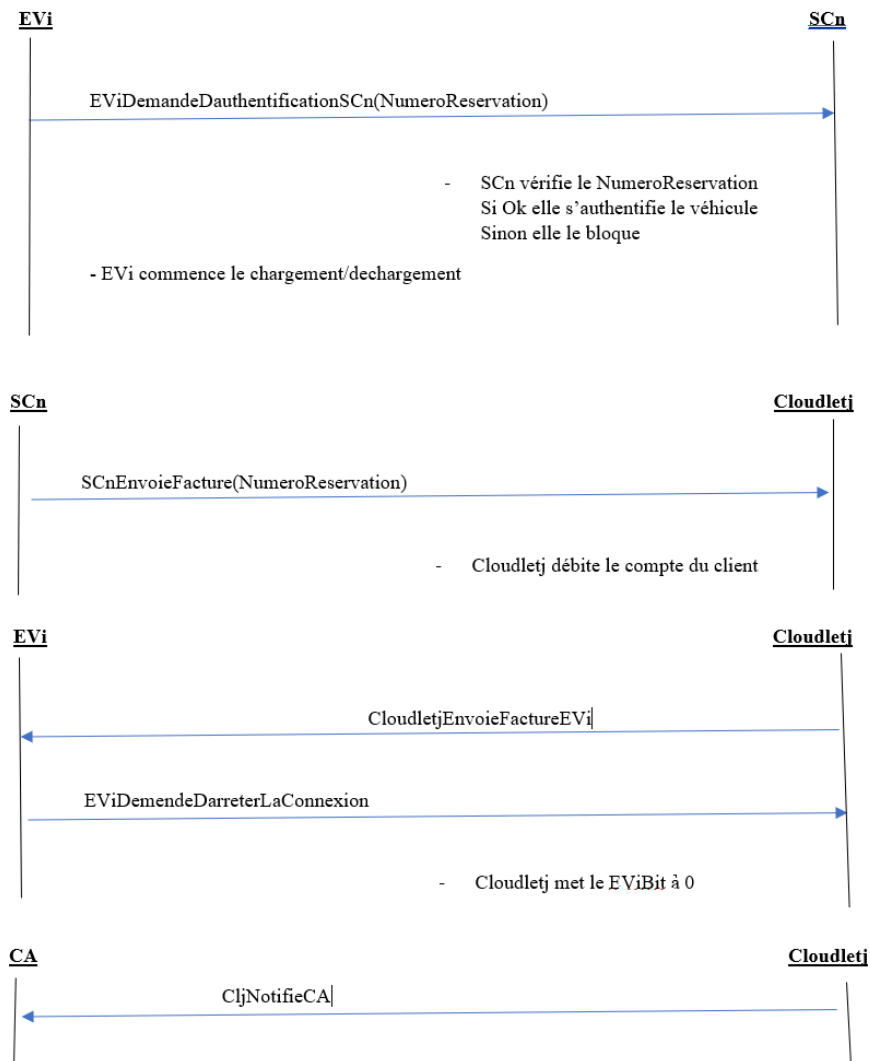
Figure 11 : Authentification mutuelle avec la SC lors du chargement/déchargement
