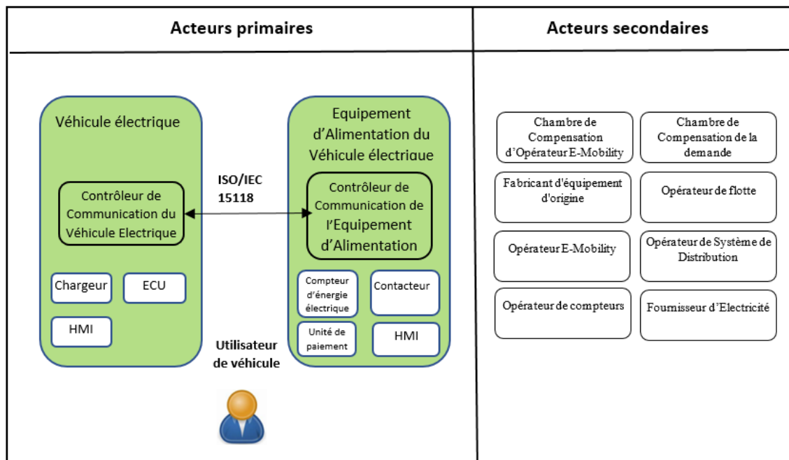
Figure 1 : Acteurs primaires et secondaires [ISO 15118-1]
